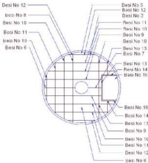
Gambar 6.5. Merakit Tutup PAH
