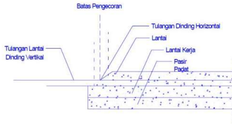
Gambar 6.3. Struktur Pengecoran Lantai Bangunan PAH
