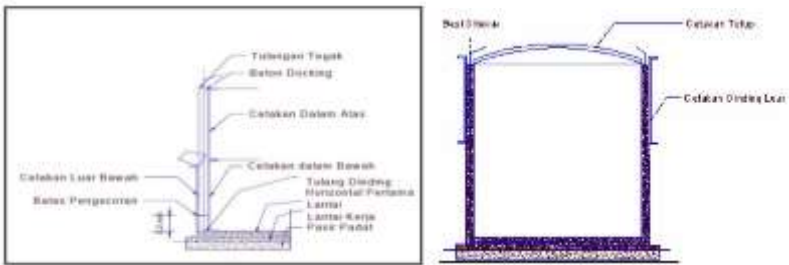
Gambar 6.4. Cetakan Luar Dinding dan Cetakan Dinding PAH
